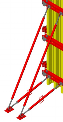
Payanda Kafası Montaj Detayı Prop Head Assembly Detail
